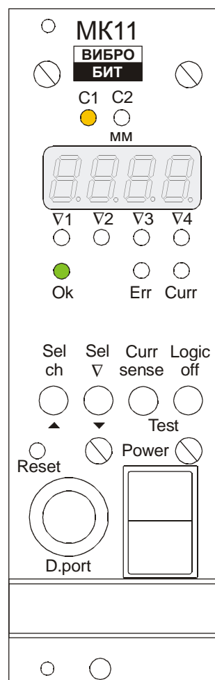
Рисунок 2 Внешний вид лицевой панели МК11-AC-11-S (ширина 40мм)
