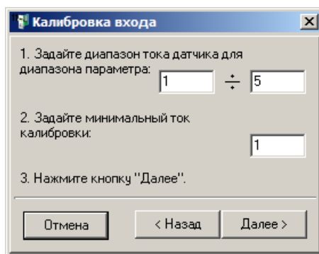
Рисунок 15. Окно калибровки входа канала измерения
