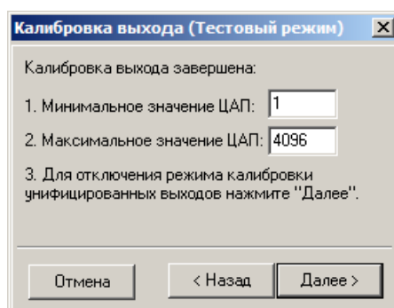
Рисунок 18. Калибровка тестового выхода (ручной режим)
