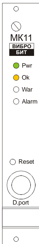
Рисунок 1. Внешний вид лицевой панели МК11-DC (ширина 20мм)
