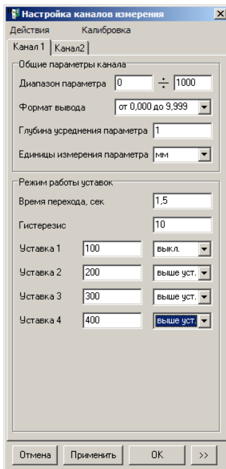
Рисунок 8. Окна настройки параметров канала измерения.
