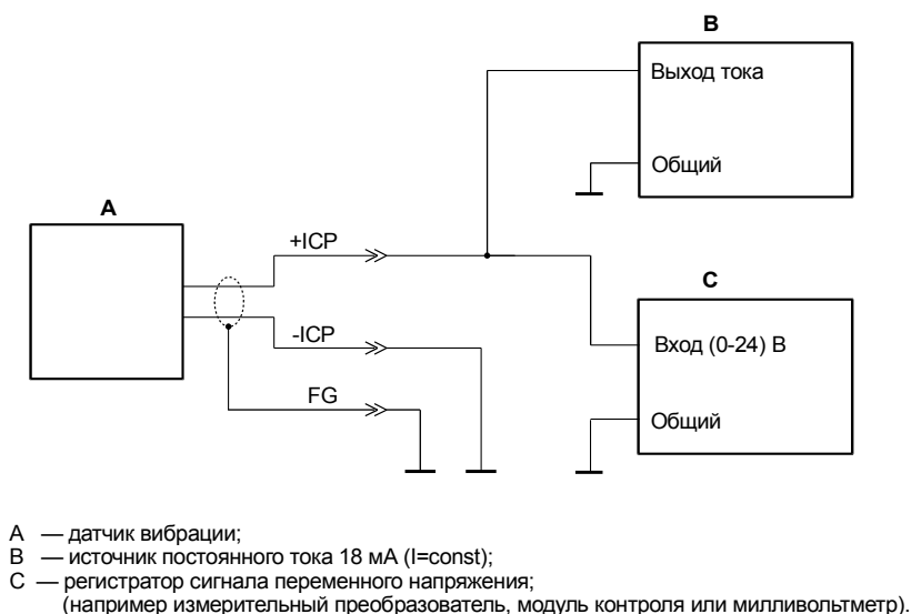
Рисунок 3 – Схема подключения датчиков типа A2xxC
