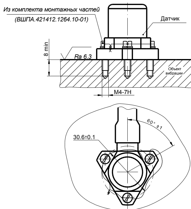
Рисунок Д.1 – Установка датчиков с корпусом типа Т3М4
