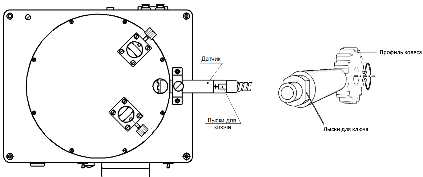
Рисунок Д.4 Установка датчиков типа «N2» и «N3» на стенде СП31
