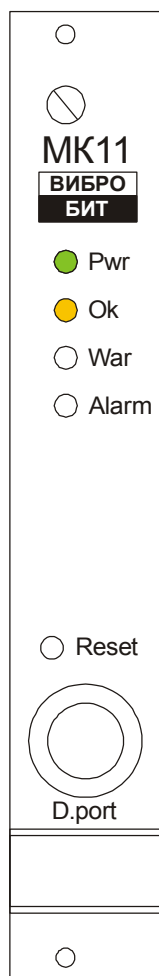
Рисунок 1. Внешний вид лицевой панели МК11-DC-R2 (ширина 20мм)
