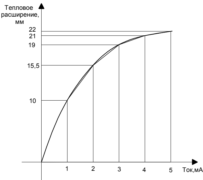
Рисунок 5. Пример характеристики датчика и таблица линеаризации
