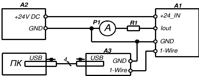
A1 - Датчик A2 - Источник питания постоянного напряжения +24 В A3 - Конвертер интерфейсов LMU400.001 R1 - Сопротивление 500± 5 % Ом P1 - миллиамперметр постоянного тока от 0 до 20 мА, КТ 0,1
