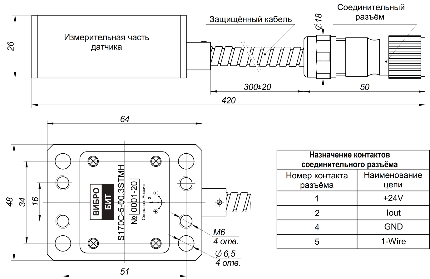
Рис. 1 — Внешний вид Датчика*
