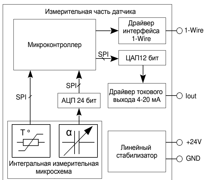
Рис. 2 Структурная схема Датчика
